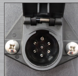
7-Way Round Pin (J560)
